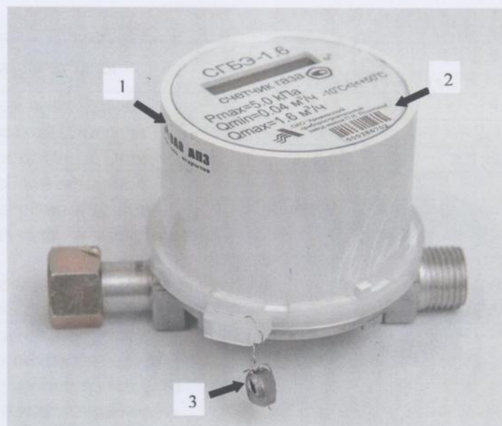
Рисунок 1 - Общий вид и схема пломбирования счётчиков газа
